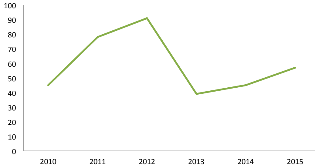
Nombre de transects suivis dans le Nord-Pas-de-Calais depuis 2010
