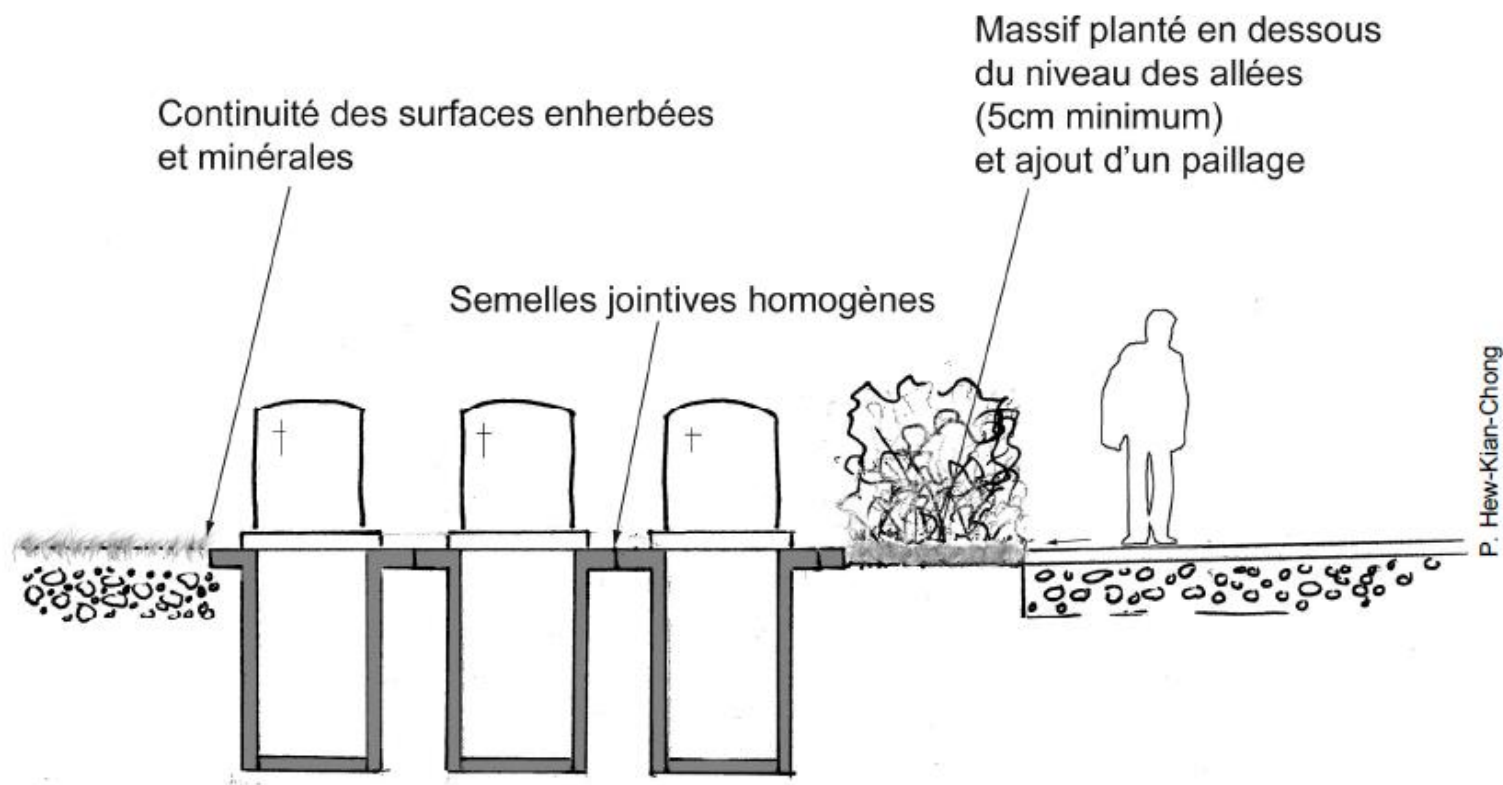
Fig. 2. Coupe de principe d'un nouvel aménagement
